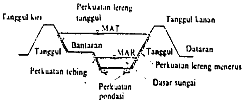
Gambar 2.1. Jenis-jenis perkuatan lereng (Dr. Ir. Suyono Sosrodarsono)
