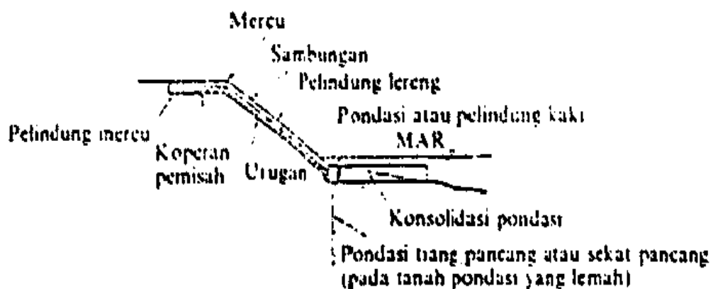
Gambar 2.2. Konstruksi perkuatan lereng (Dr. Ir. Suyono Sosrodarsono)
