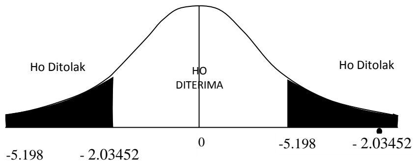
Gambar 5.5 Kurva Akuntabilitas
