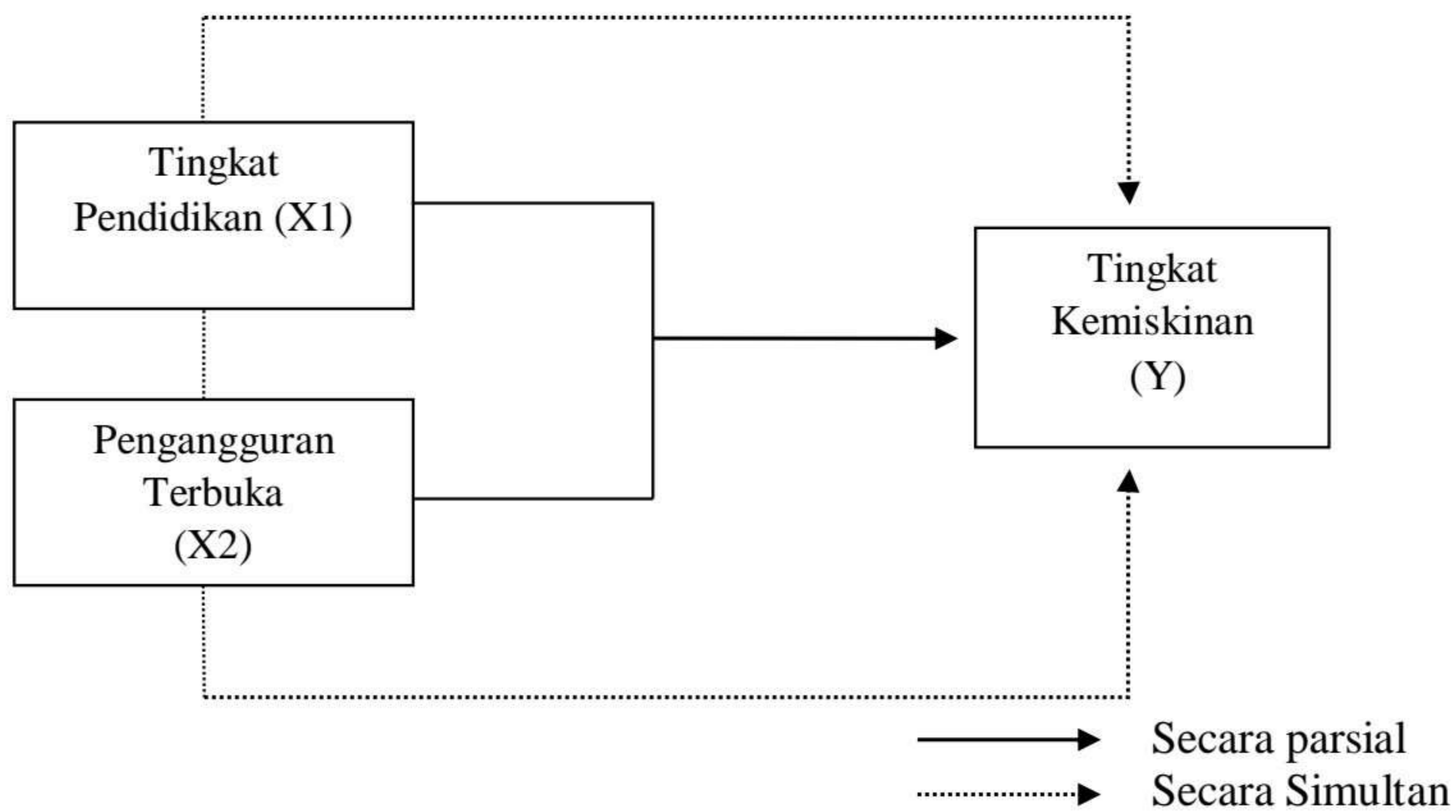
Gambar 2.2 Kerangka Pikir
