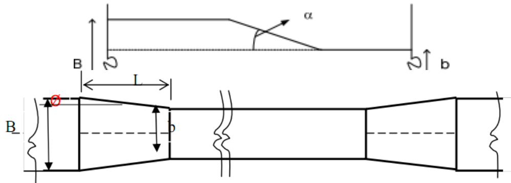
Gambar 2.1 Panjang Peralihan dan Transisi pada Talang
