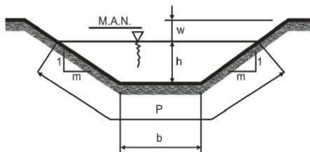
Gambar 2.3 Saluran Trapesium
